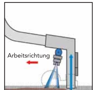
Funktionsweise der Sprühextraktion
