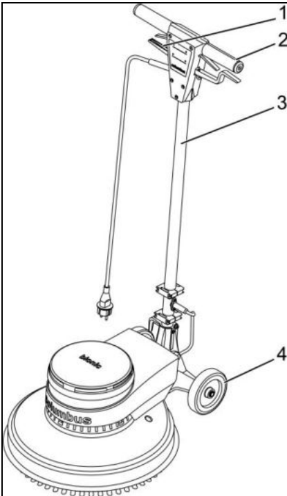
Fig. 13 : Ajustage du manche de guidage
