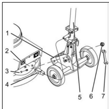
Fig. 5 : Montage du manche de guidage
