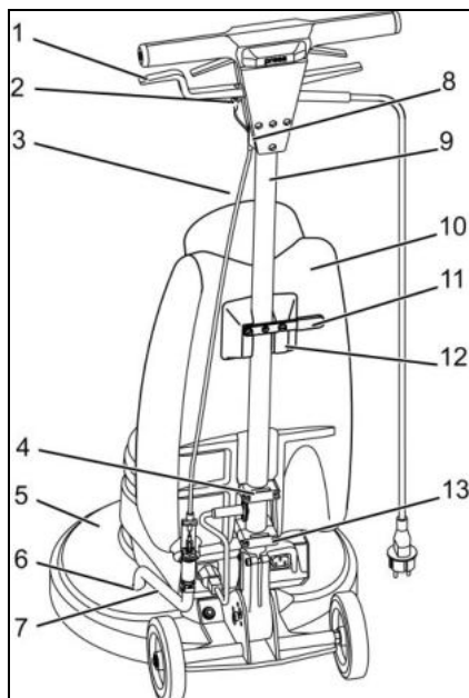
Fig. 8 : Montage du réservoir
