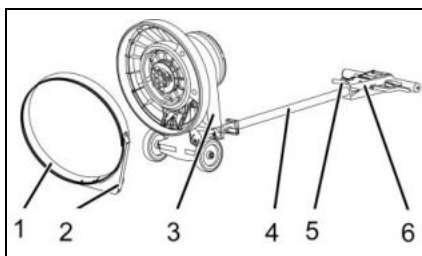
Fig. 10 : Montage de l'appareil d'aspiration
