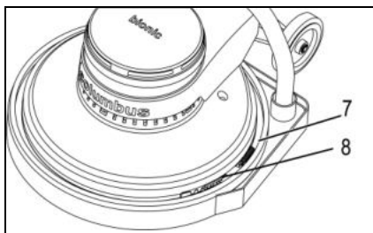
Fig. 11: Montage de l'anneau d'aspiration
