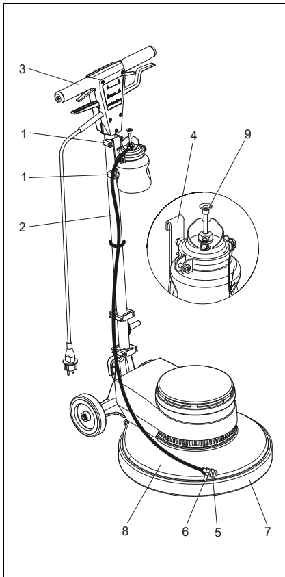
Fig. 7 : Montage du pulvérisateur
