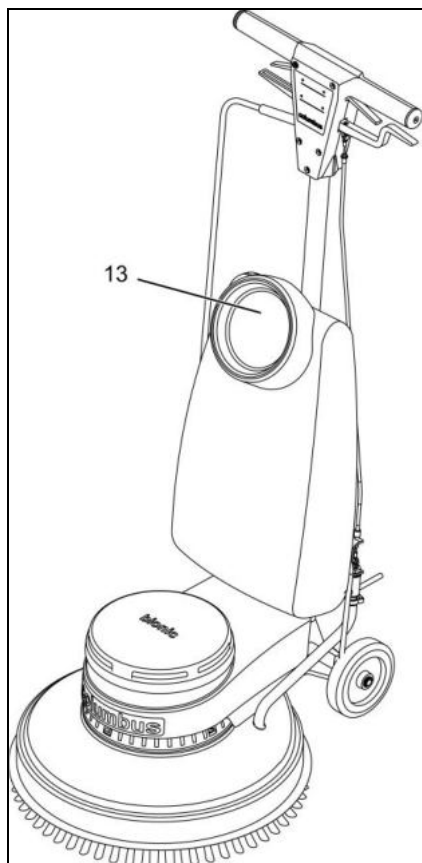
Fig. 9 : Remplissage du réservoir
