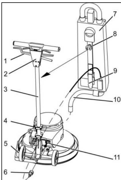
Fig. 12 : Montage du récipient d'aspiration
