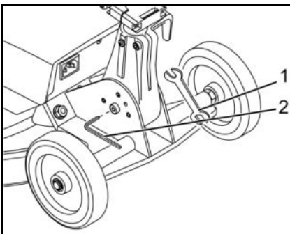
Fig. 14 : Ajustage de la charnière pivotante
