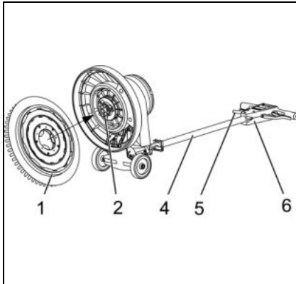
Fig. 16 : Montage manuel de l'accessoire de nettoyage
