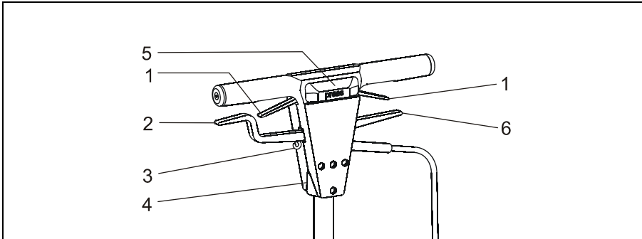
Abb. : Führungsriff
