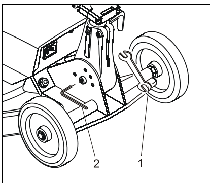
Abb. : Drehgelenk einstellen
