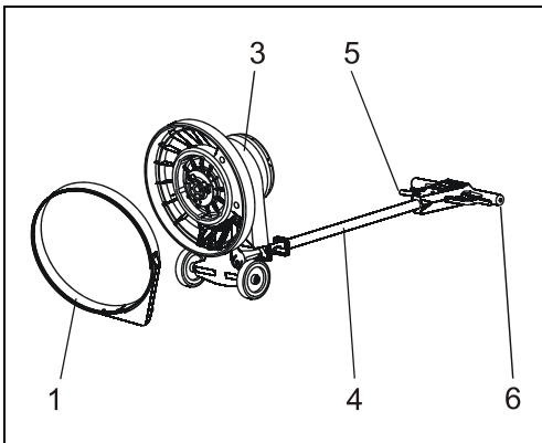
Abb. : Absaugung montieren
