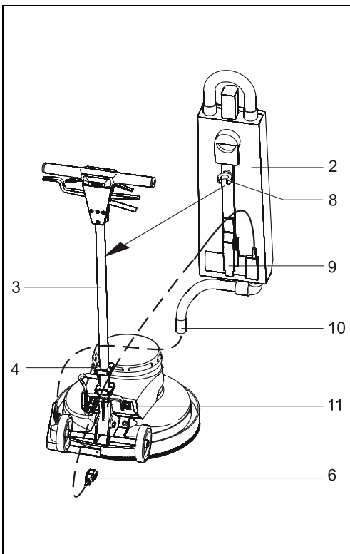
Abb. : Saugbehälter montieren
