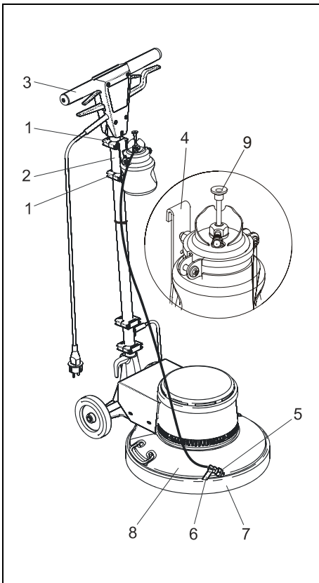
Abb. .. Sprühgerät montieren
