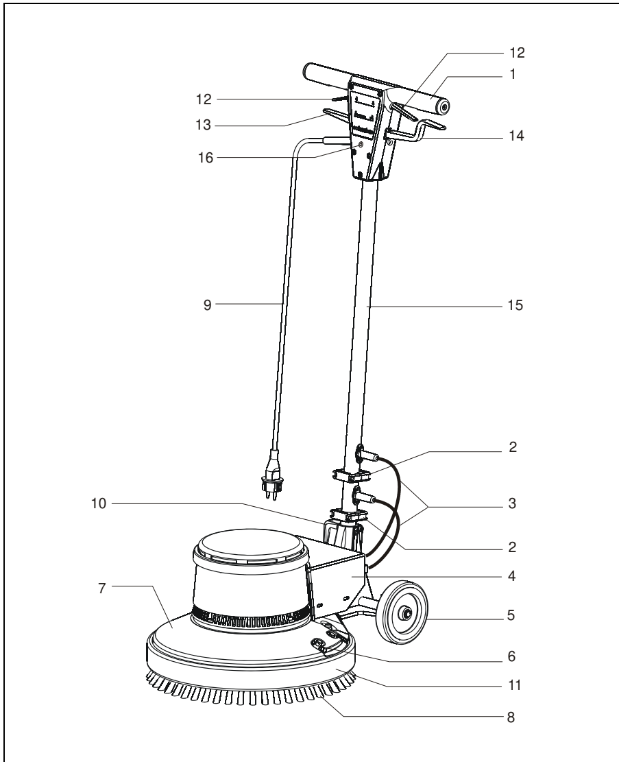
Abb. .. Geräteübersicht
