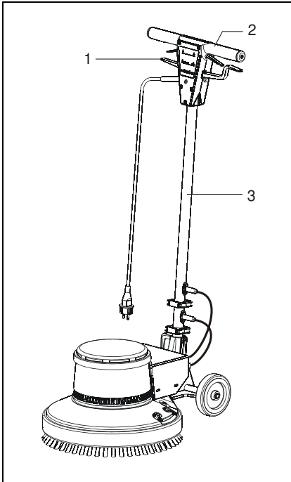
Abb. : Führungsstange einstellen
