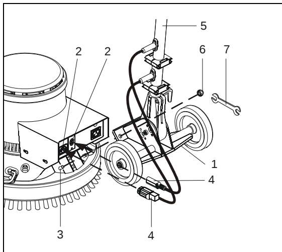
Fig. . : Montage du manche de guidage
