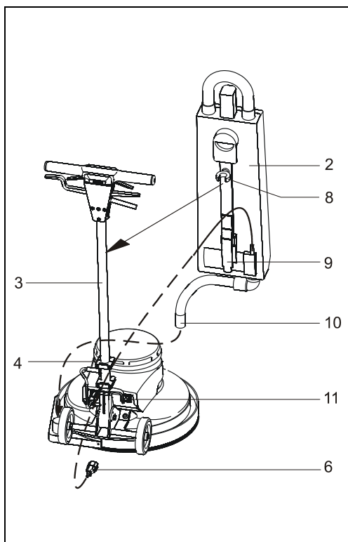
Fig.. : Montage du récipient d'aspiration
