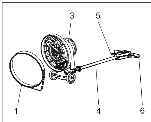
Fig. . : Montage de l'appareil d'aspiration
