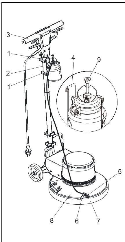
Fig. .: Montage du pulvérisateur
