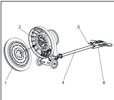
Fig. . : Montage manuel de l'accessoire de nettoyage
