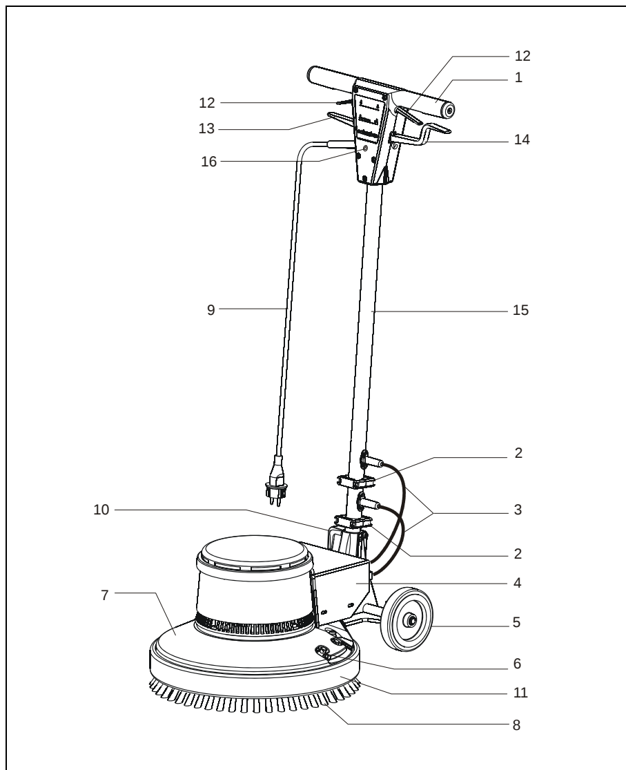
Fig.. : Vue d'ensemble de l'appareil
