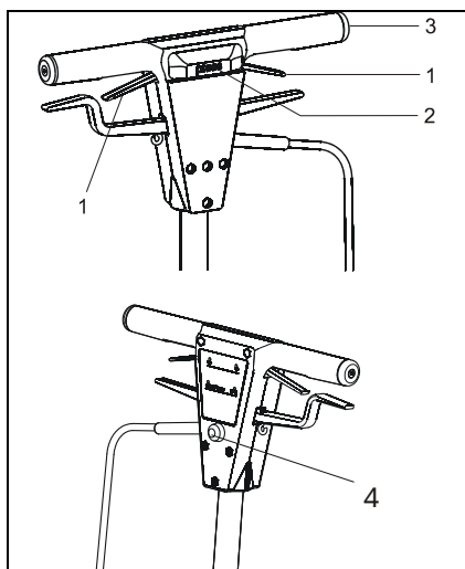
Fig. . : Mise en marche et arrêt
