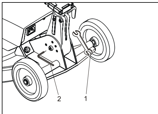
Fig. . : Ajustage de la charnière pivotante
