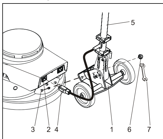
Fig. . : Montage du manche de guidage
