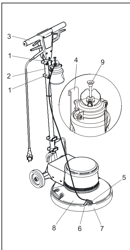
Fig. .: Montage du pulvérisateur
