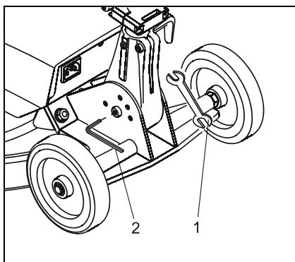
Fig. . : Ajustage de la charnière pivotante
