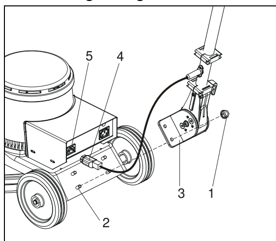
Abb. 5: Führungsstange montieren
