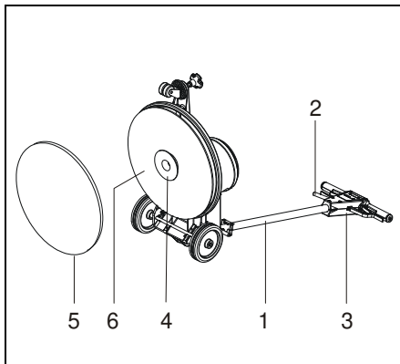
Abb. 14: Pad einsetzen
