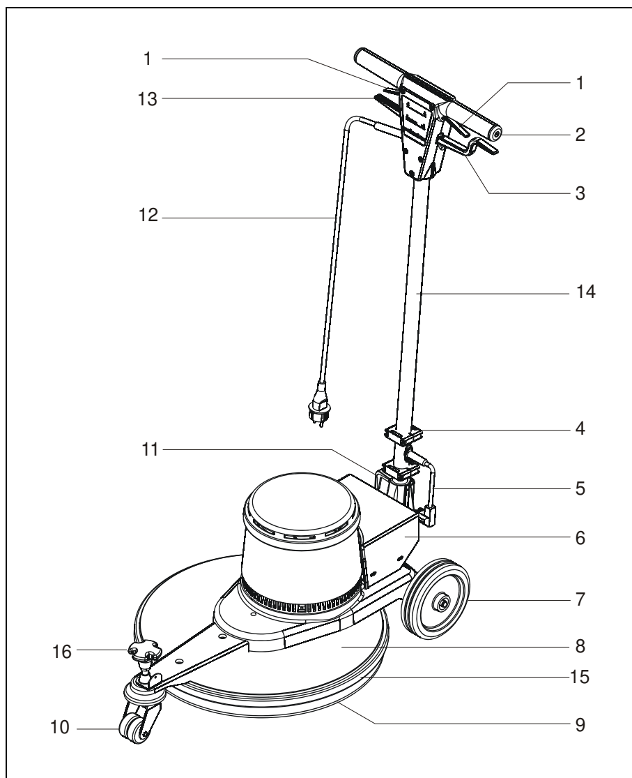
Abb. 1: Geräteübersicht
