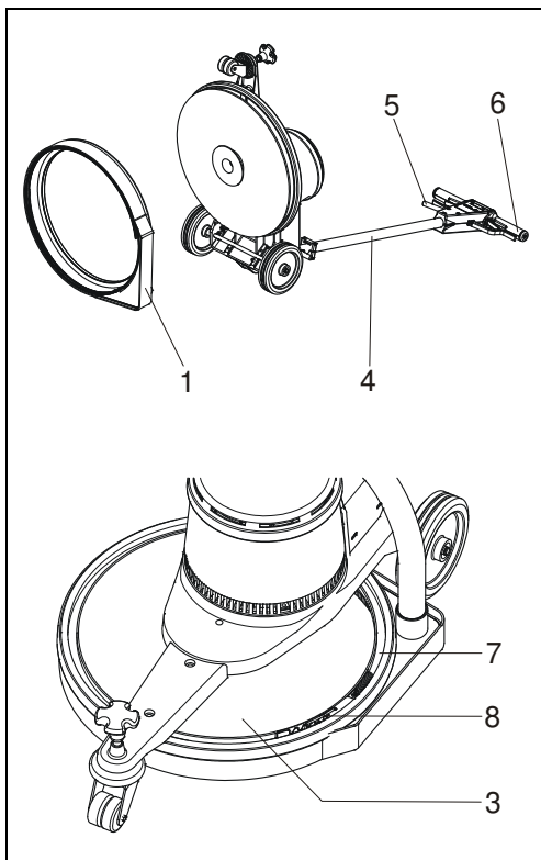
Abb. 8: Absaugring montieren
