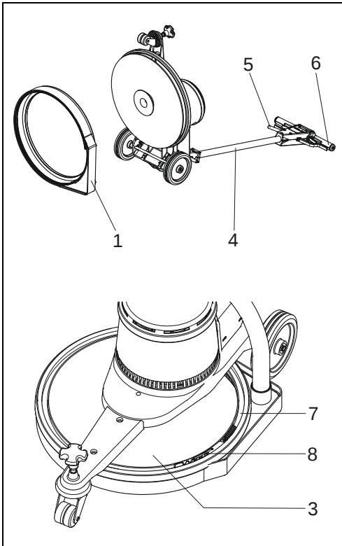
Fig. 8 : Montage de l'appareil d'aspiration
