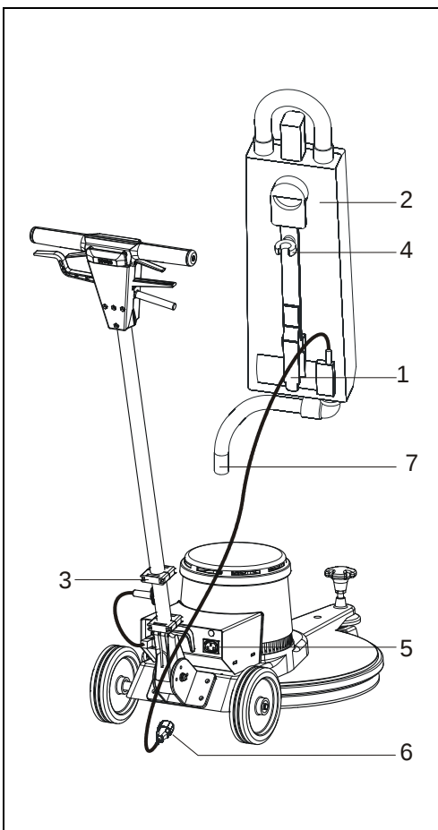
Fig.9 : Montage du récipient d'aspiration
