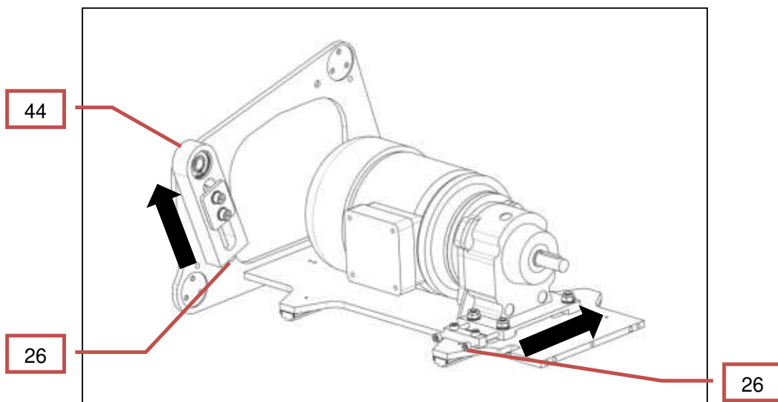
Imagen 23: Tensar las cadenas
