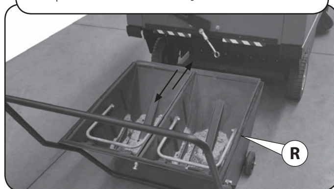
[AKS 85|BM 120 Performance] Machine avec vidange manuelle du conteneur des ordures
