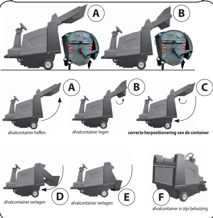
[AKS 85]BM 150H Performance] Machine met hydraulische afvoer van de afvalcontainer
