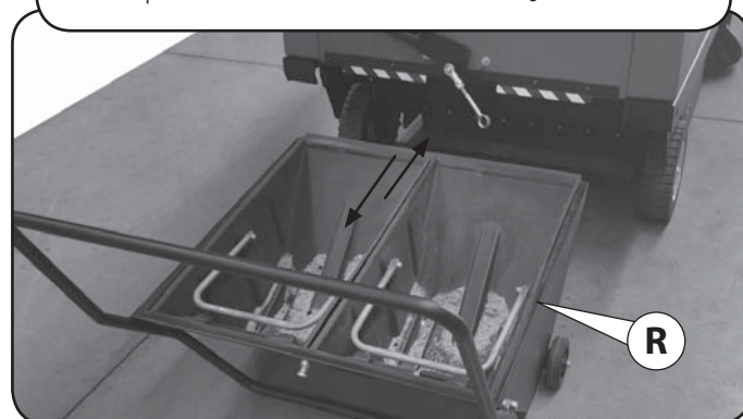
[AKS 85|BM 120 Performance] Maschine mit manueller Entleerung des Abfallbehälters
