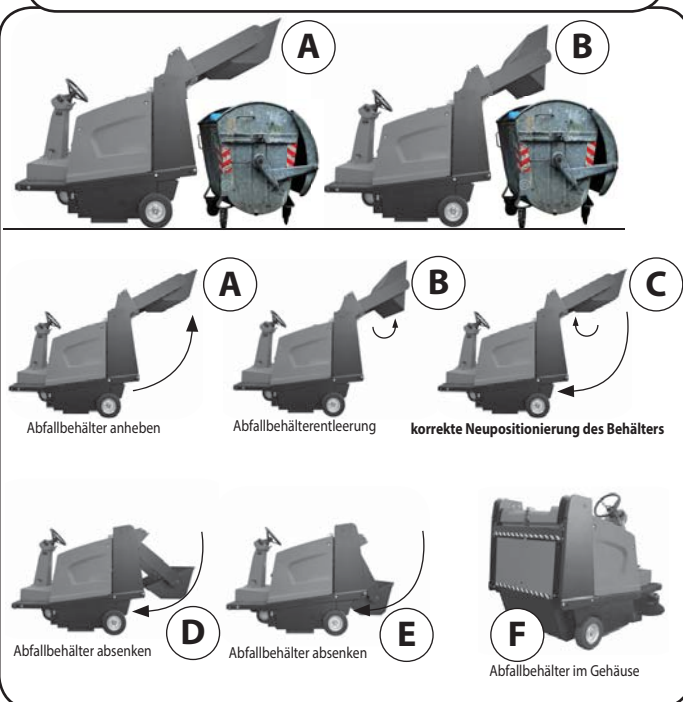
[AKS 85|BM 150H Performance] Maschine mit hydraulischer Entleerung des Abfallbehälters
