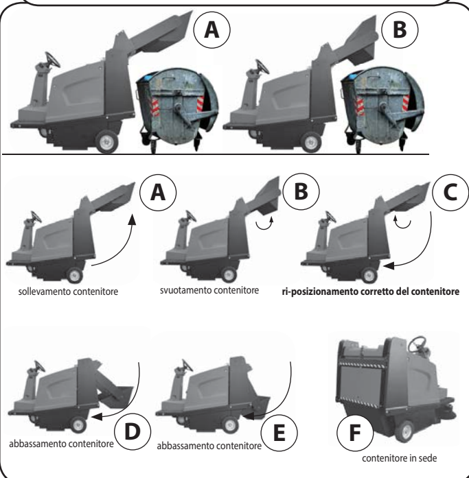
[AKS 85|BM 150H Performance] Macchina con scarico idraulico del contenitore rifiuti
