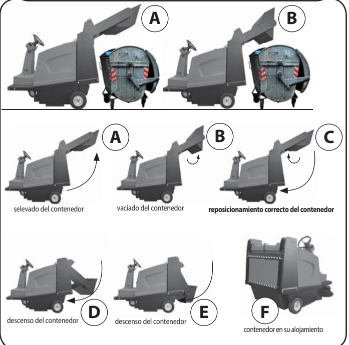
[AKS 85]BM 150H Performance] Máquina con vaciado hidráulico del contenedor de basura
